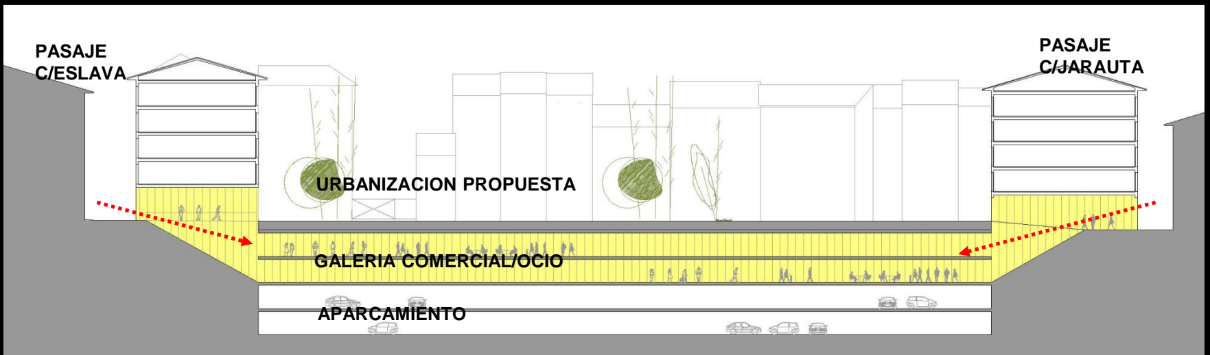
SECCION LONGITUDINAL GALERIA COMERCIAL Y DE OCIO.
